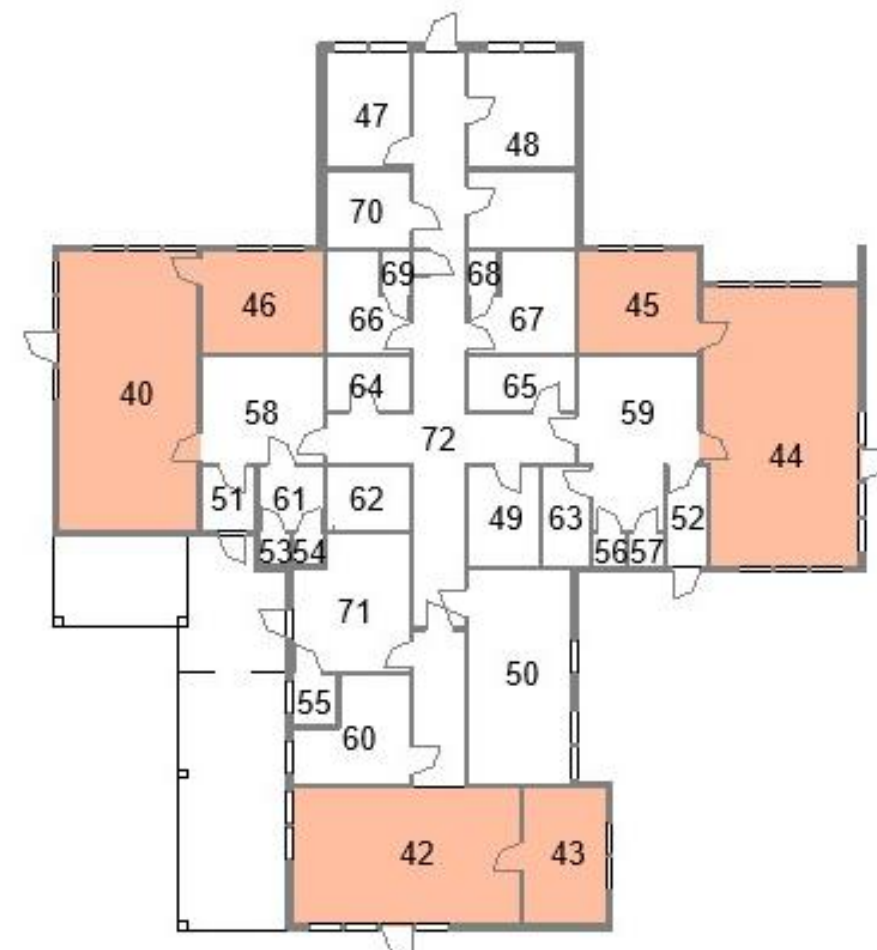
Figur 6 LOA på Leabøen barnehage etter oppgradering
