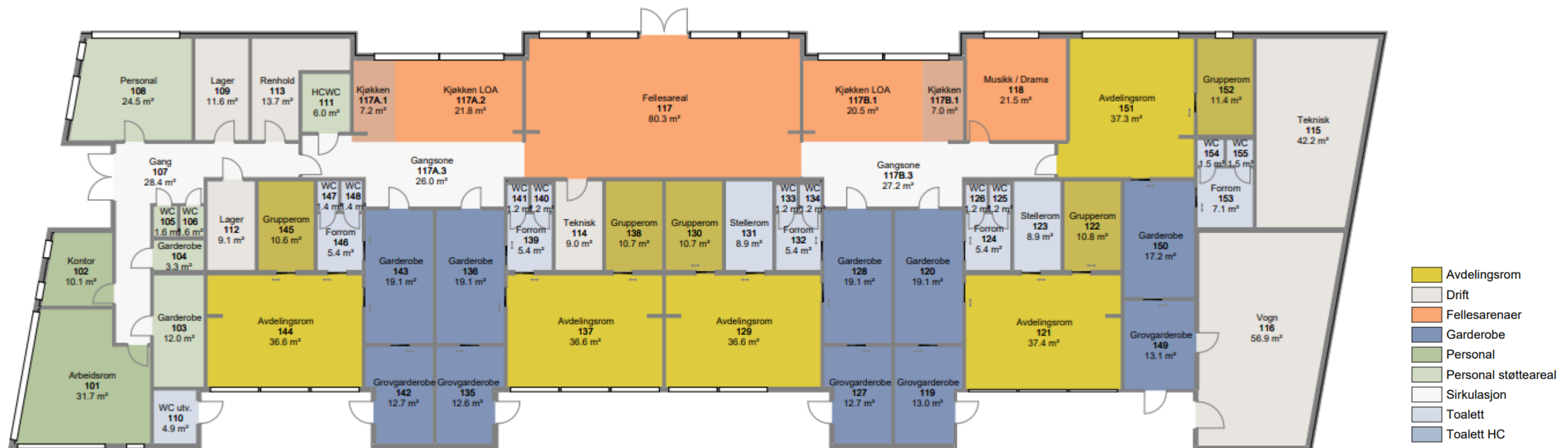
Figur 3: Plantegning Veslefrikk barnehage med funksjoner
